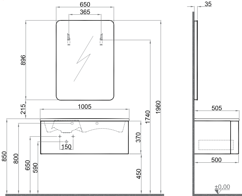
100 cm Sağ Etajerli Lavabolu Dolap Ön ve Yan Görünüş
