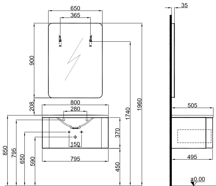
80 cm Lavabolu Dolap Ön ve Yan Görünüş
