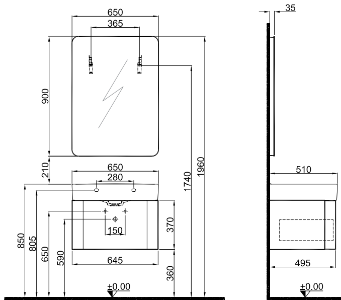
65 cm Lavabolu Dolap Ön ve Yan Görünüş
