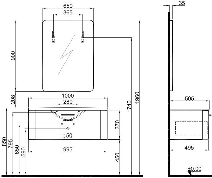
100 cm Lavabolu Dolap Ön ve Yan Görünüş
