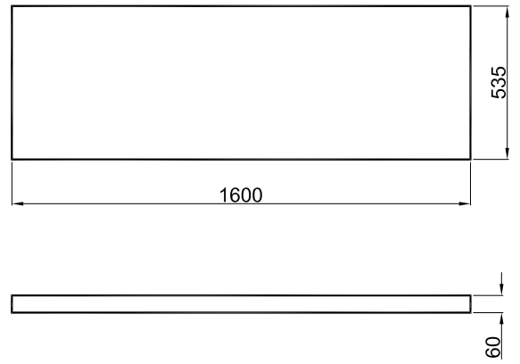
160 cm Raf Ön ve Yan Görünüş
