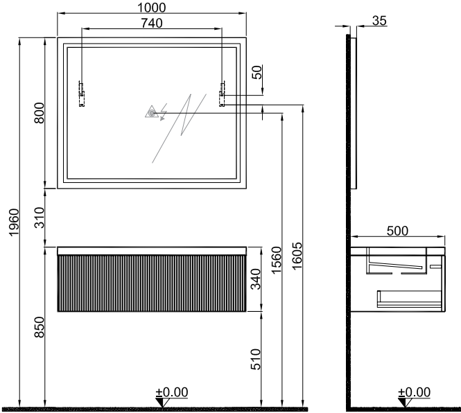
100 cm Lavabolu Dolap Ön ve Yan Görünüş
