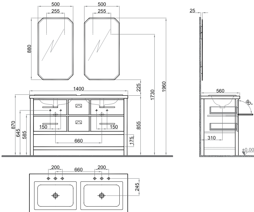
140 cm Lavabolu Dolap Ön ve Yan Görünüş
